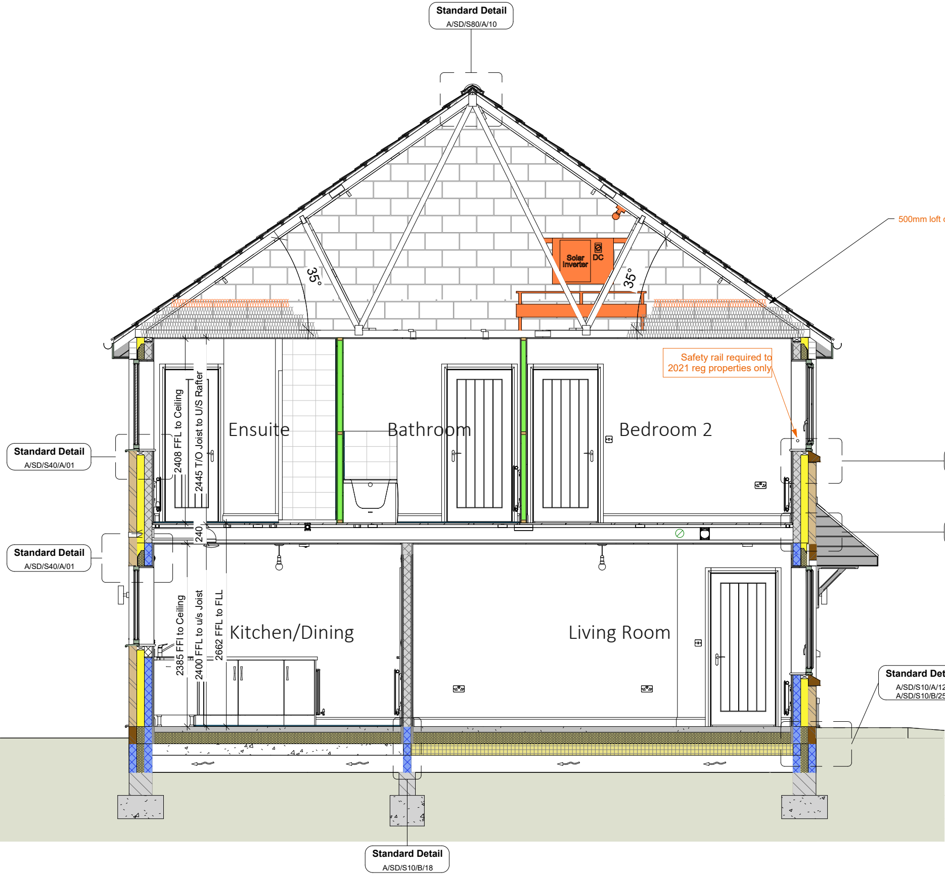
A Section A - A 1 : 50
